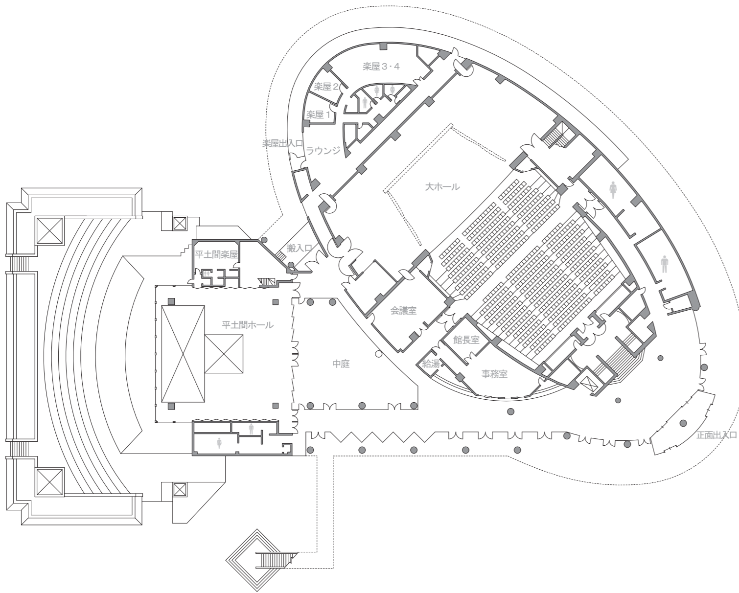
1階平面図
